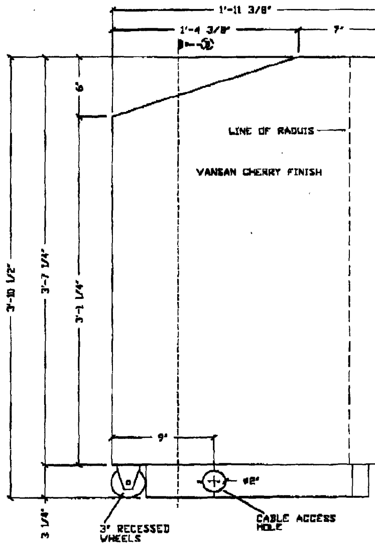
END ELEVATION
